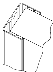
PD-3, 4 og 5 Aluminiumskarm Fast karm for vegttykkelser PD-3: 75 mm PD-4: 80 mm PD-5: 100 mm
