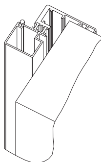
KL-2 Aluminiumskarm m/brutt kuldebro Fast karm for veggtykkelser fortrinnsvis over 300 mm
