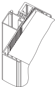
KL-1 Aluminiumskarm m/brutt kuldebro Helomsluttende justerbar karm for veggtykkelser fra 70 til 300 mm
