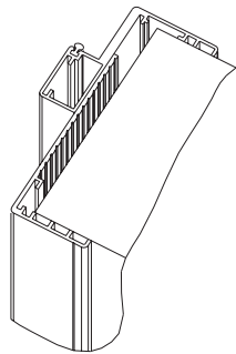
IL-1 Aluminiumskarm Helomsluttende justerbar karm for veggtykkelser fra 70 til 300 mm
