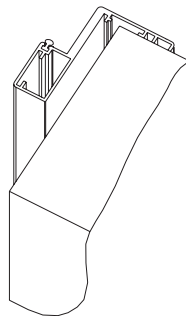
IL-2 Aluminiumskarm Fast karm for veggtykkelser fortrinnsvis over 300 mm
